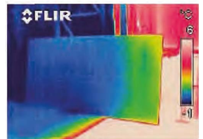
Airdoor ingeschakeld
