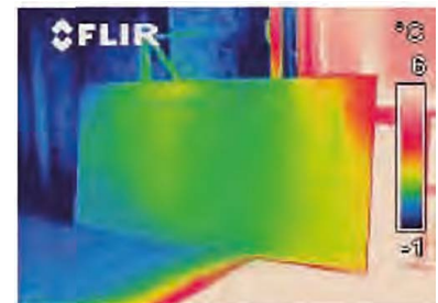
Airdoor uitgeschakeld
